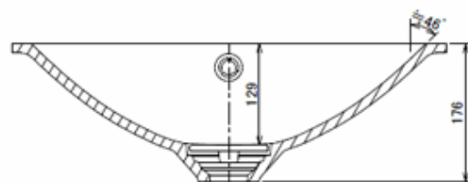
A-A 断面図
